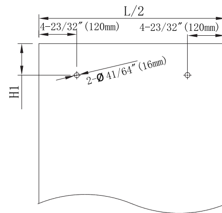
Corte en el fijo de cristal
