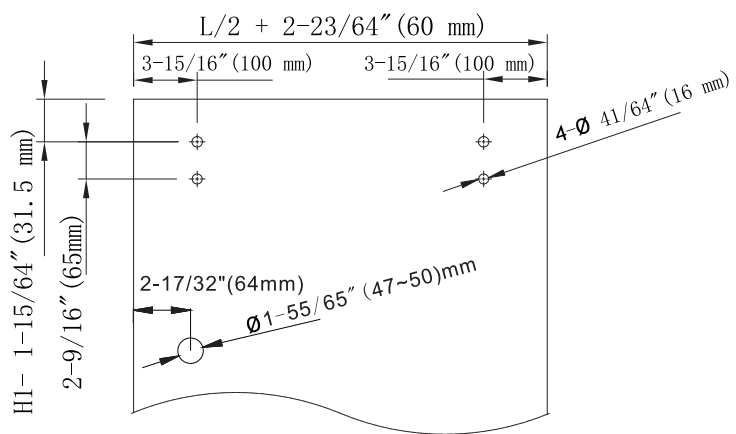
Corte en la puerta de cristal
